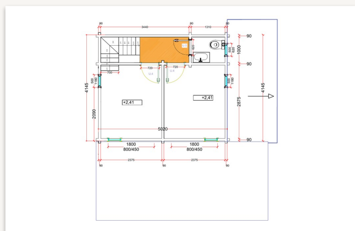
Plan étage (mansarde)
