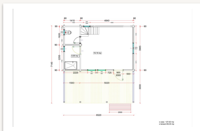
Plan rez-de-chaussée
